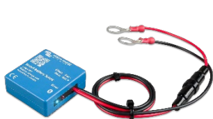
Smart Battery Sense Permite la carga con compensación de temperatura y tensión.
